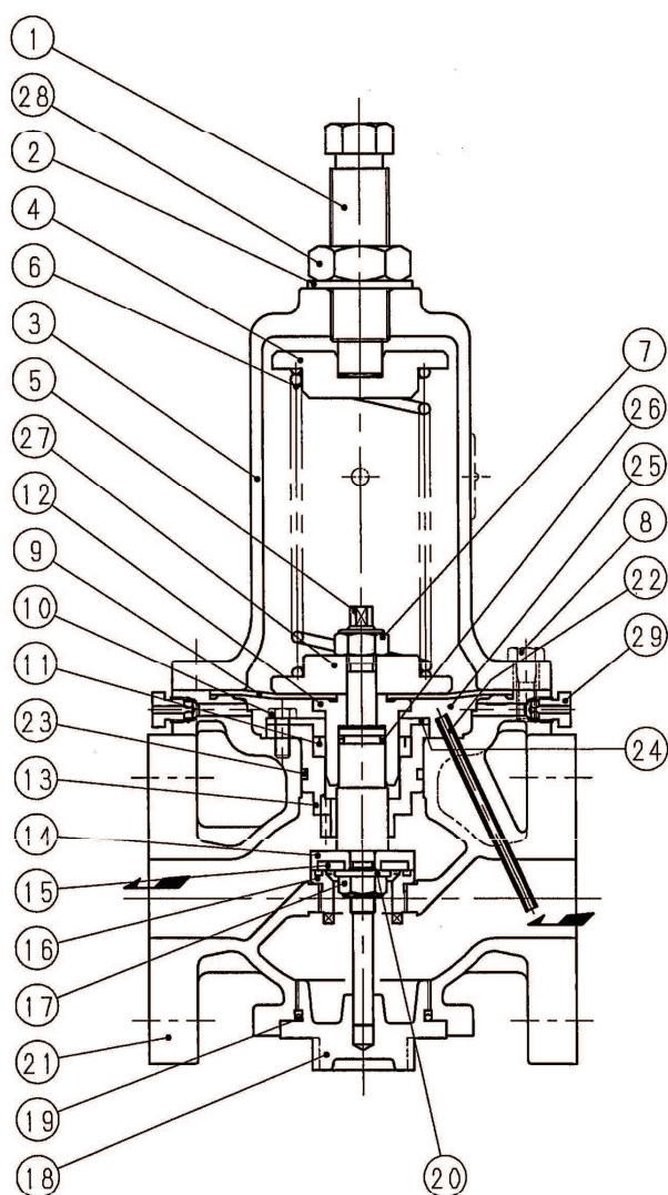
図1 構造図 呼び径(15~50A)
