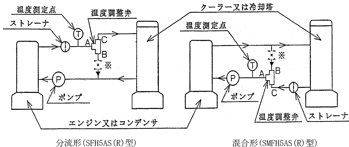
図3 標準的配管例
