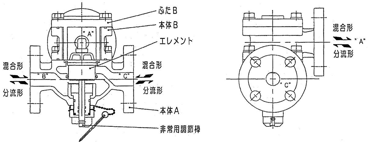
図1 構造図
