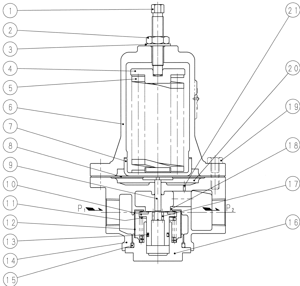
図1 構造図
