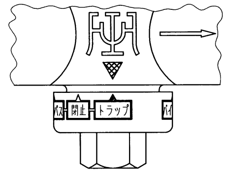
切換部外觀図
