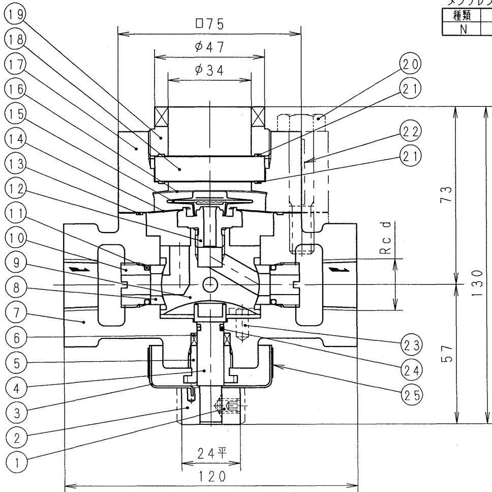
切換部外観図
