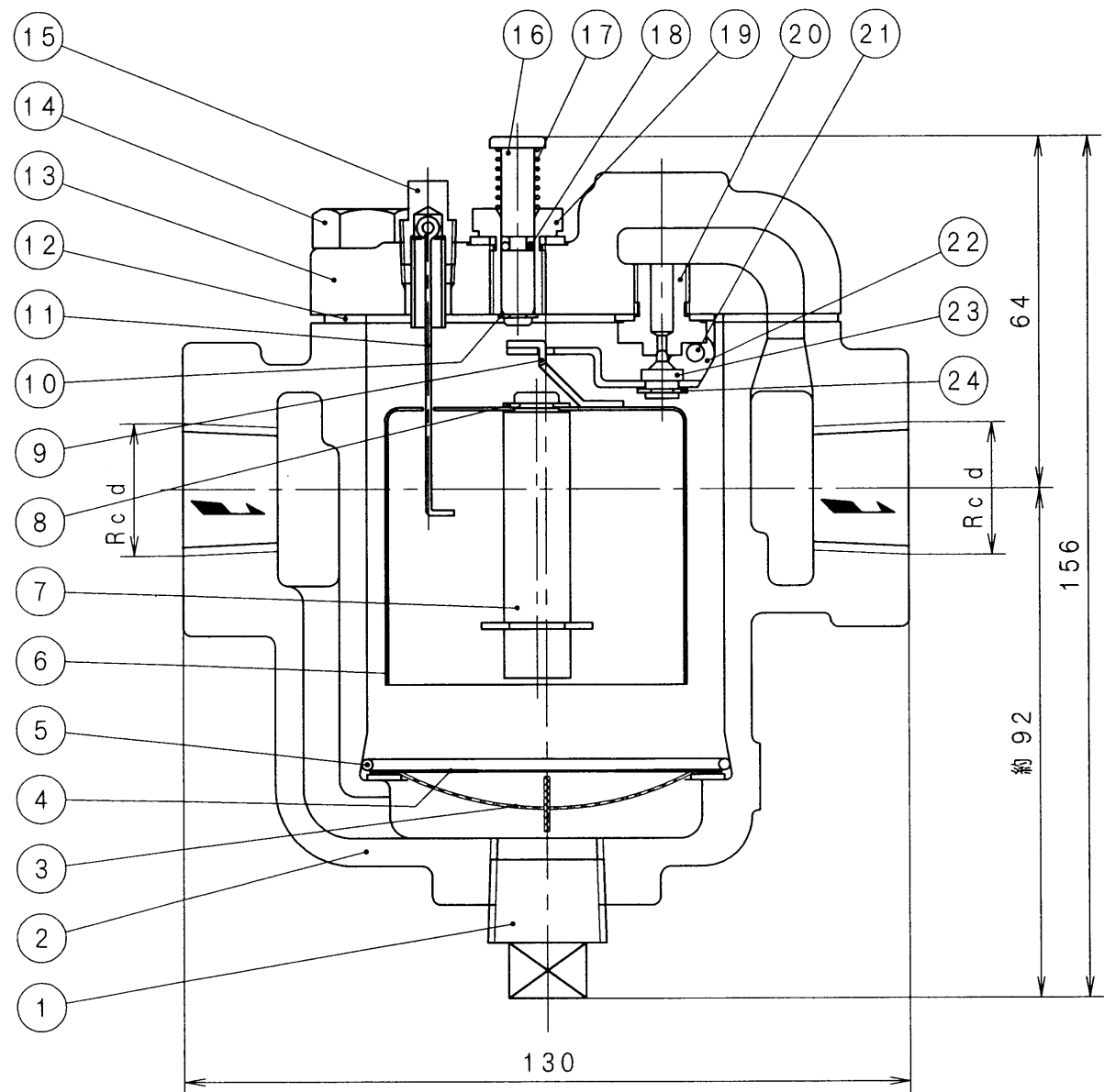
本図ハ閉弁状態ヲ示マス。
