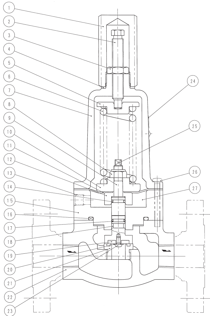
図1 RPD52-2型背圧弁
